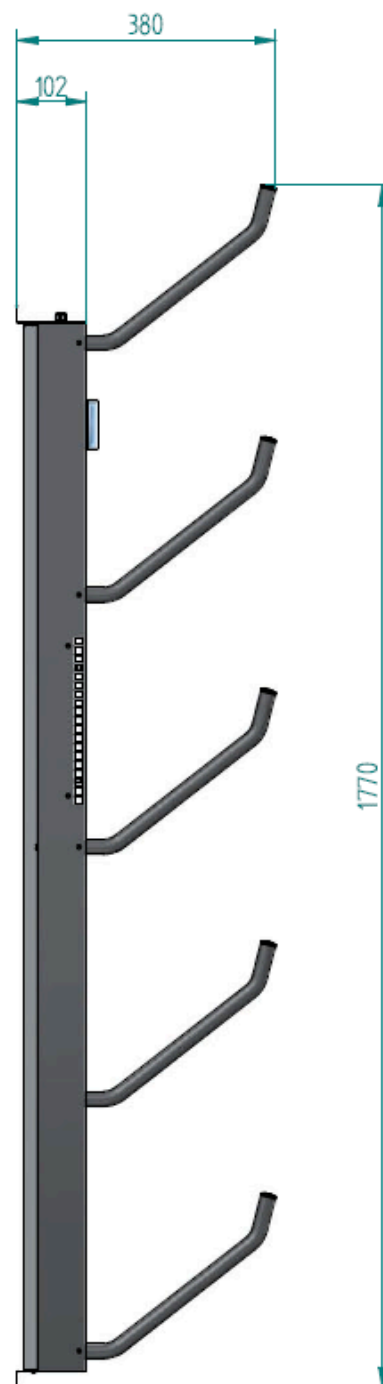
VISTA LATERALE
